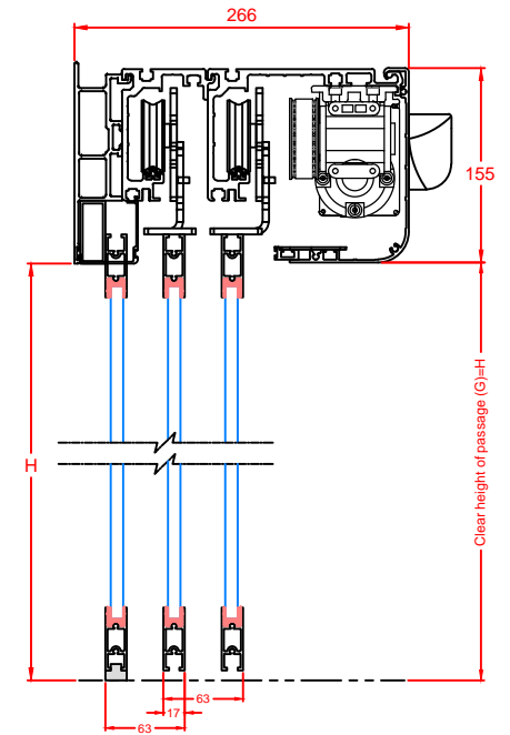
Section A-A
